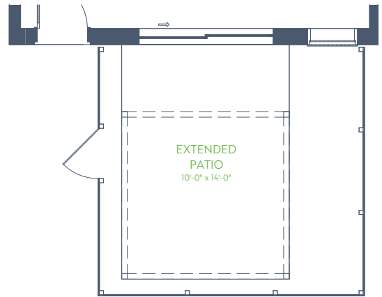
OPTIONAL EXTENDED PATIO + OPTIONAL EXTENDED TRELLIS
